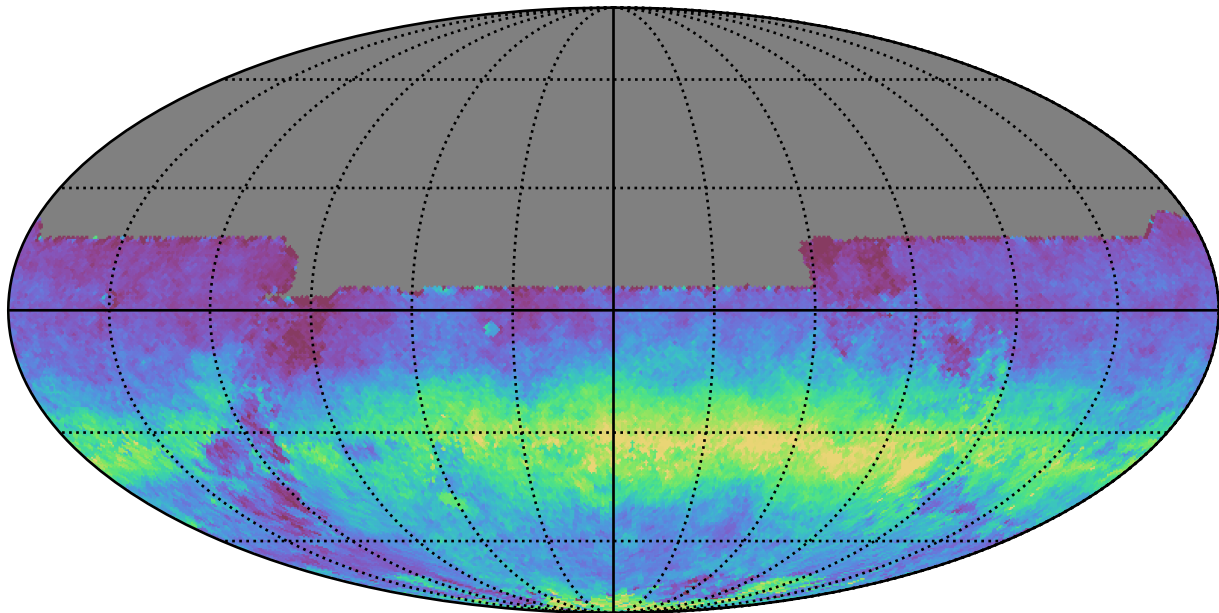
baseline_v3.2_10yrs All sky y band: AngleRms rotSkyPos
