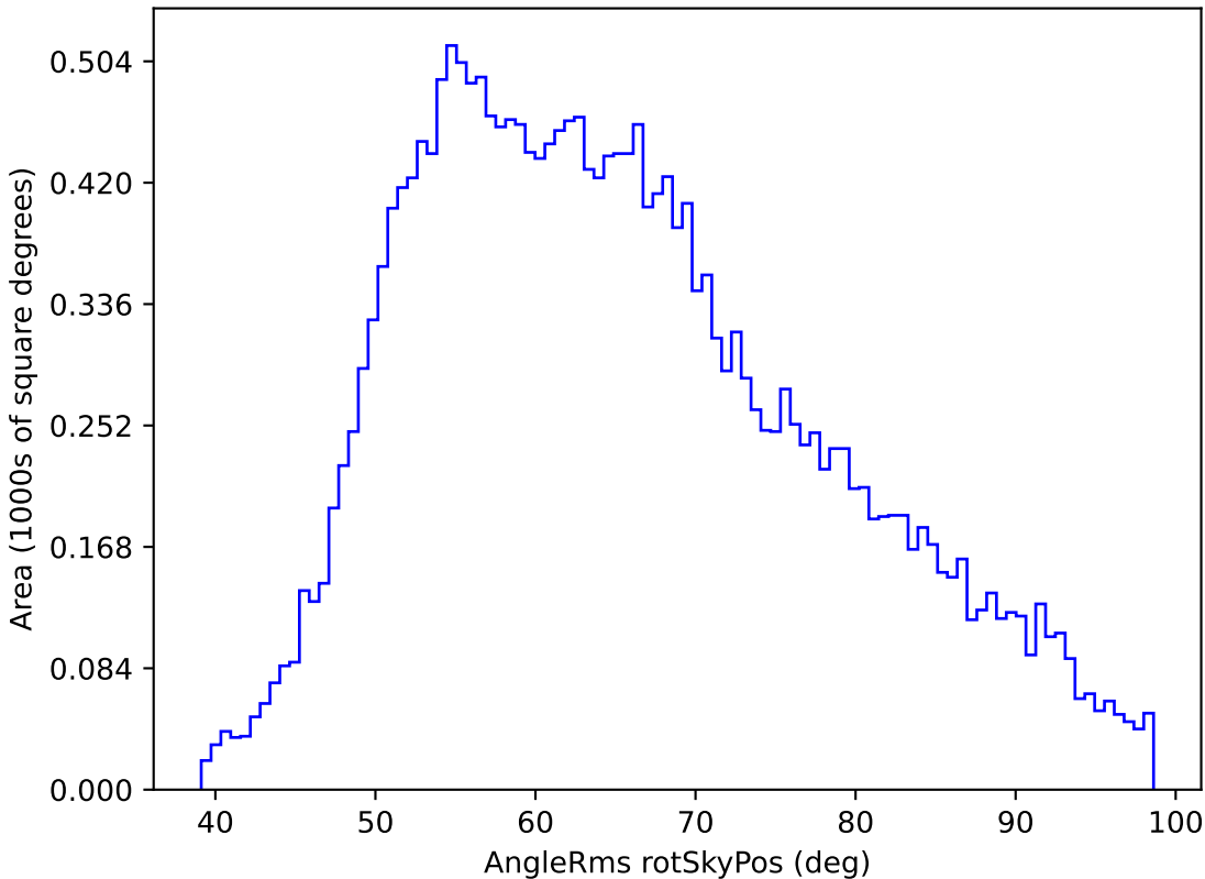
baseline_v3.2_10yrs All sky y band: AngleRms rotSkyPos
