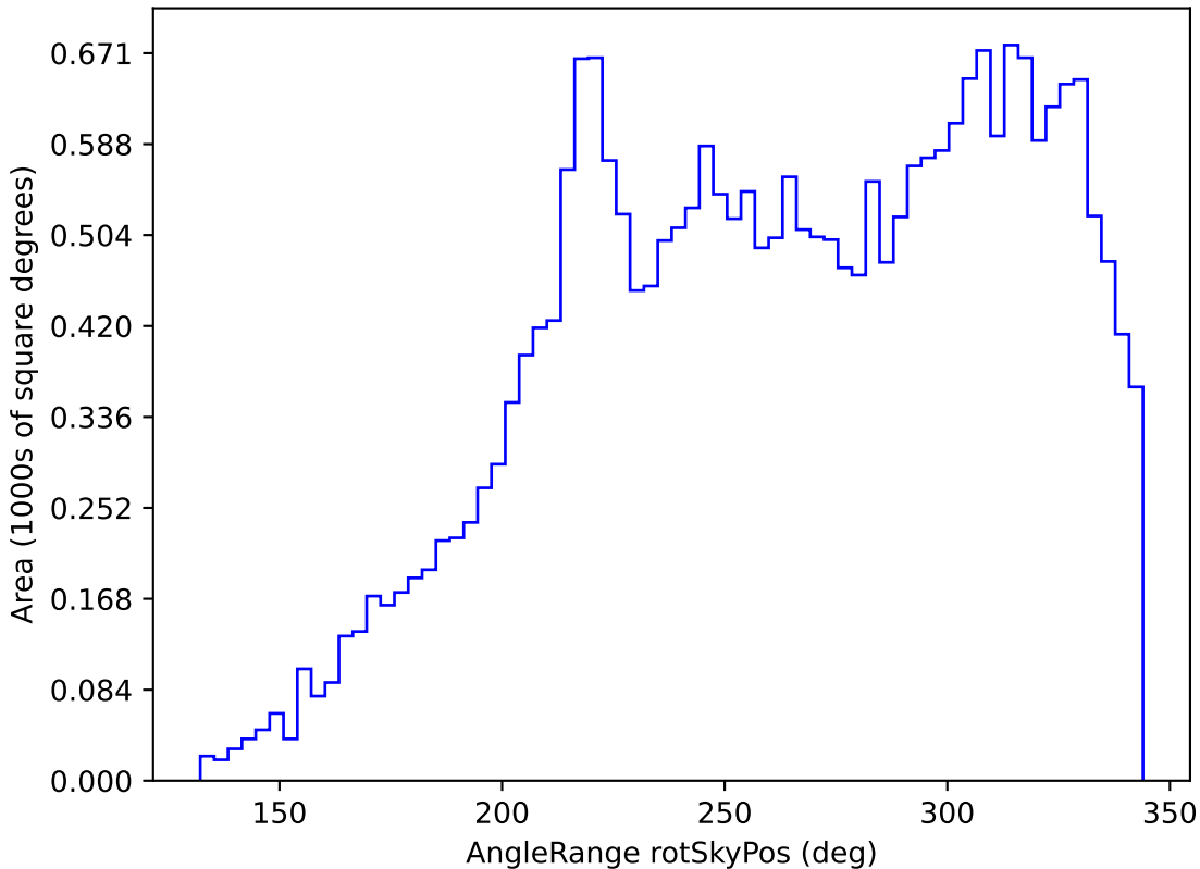
baseline_v3.2_10yrs All sky z band: AngleRange rotSkyPos
