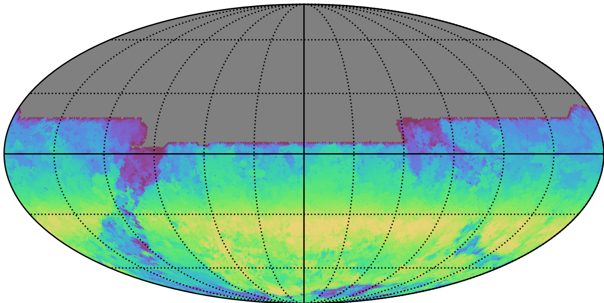
baseline_v3.2_10yrs All sky y band: AngleRange rotSkyPos
