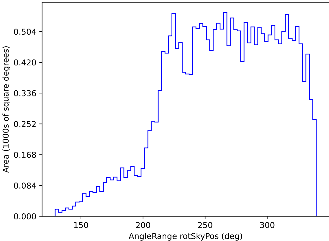
baseline_v3.2_10yrs All sky y band: AngleRange rotSkyPos
