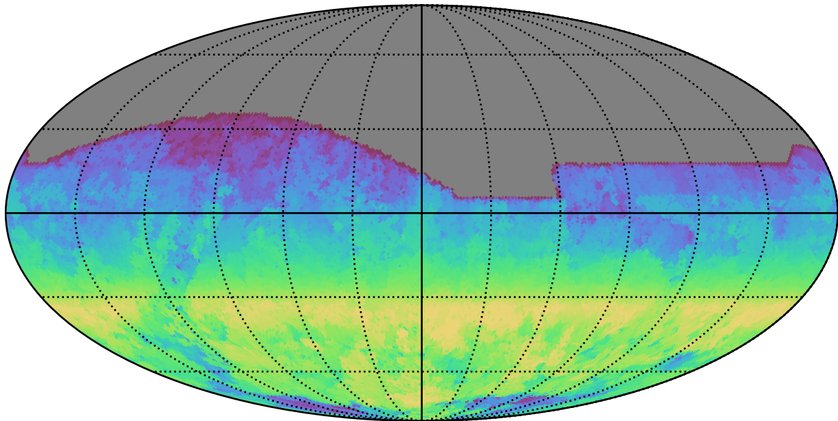
baseline_v3.2_10yrs All sky i band: AngleRange rotSkyPos
