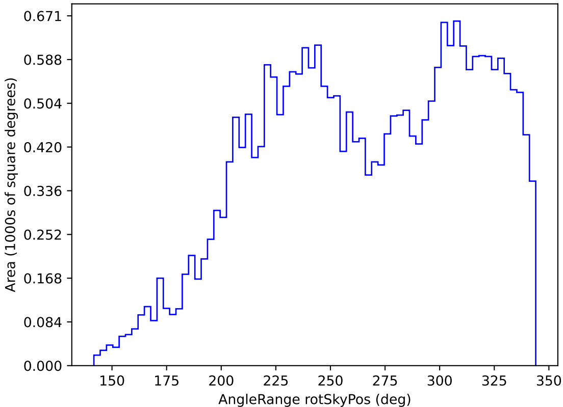
baseline_v3.2_10yrs All sky i band: AngleRange rotSkyPos
