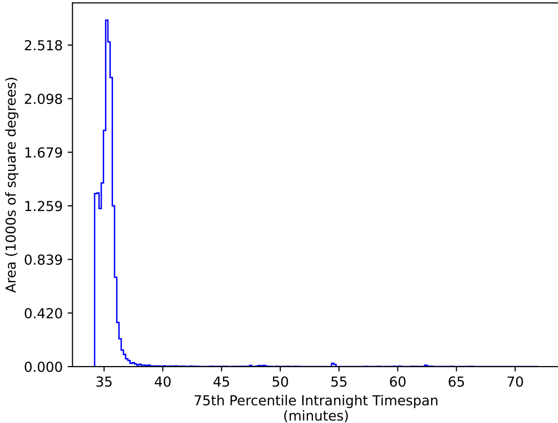
baseline_v3.2_10yrs WFD iz bands: 75th Percentile Intranight Timespan
