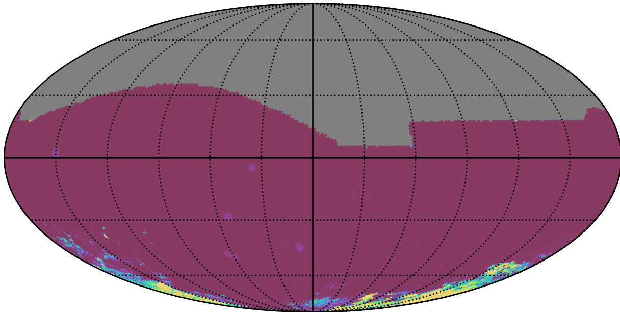
baseline_v3.2_10yrs All sky iz bands: 75th Percentile Intranight Timespan
