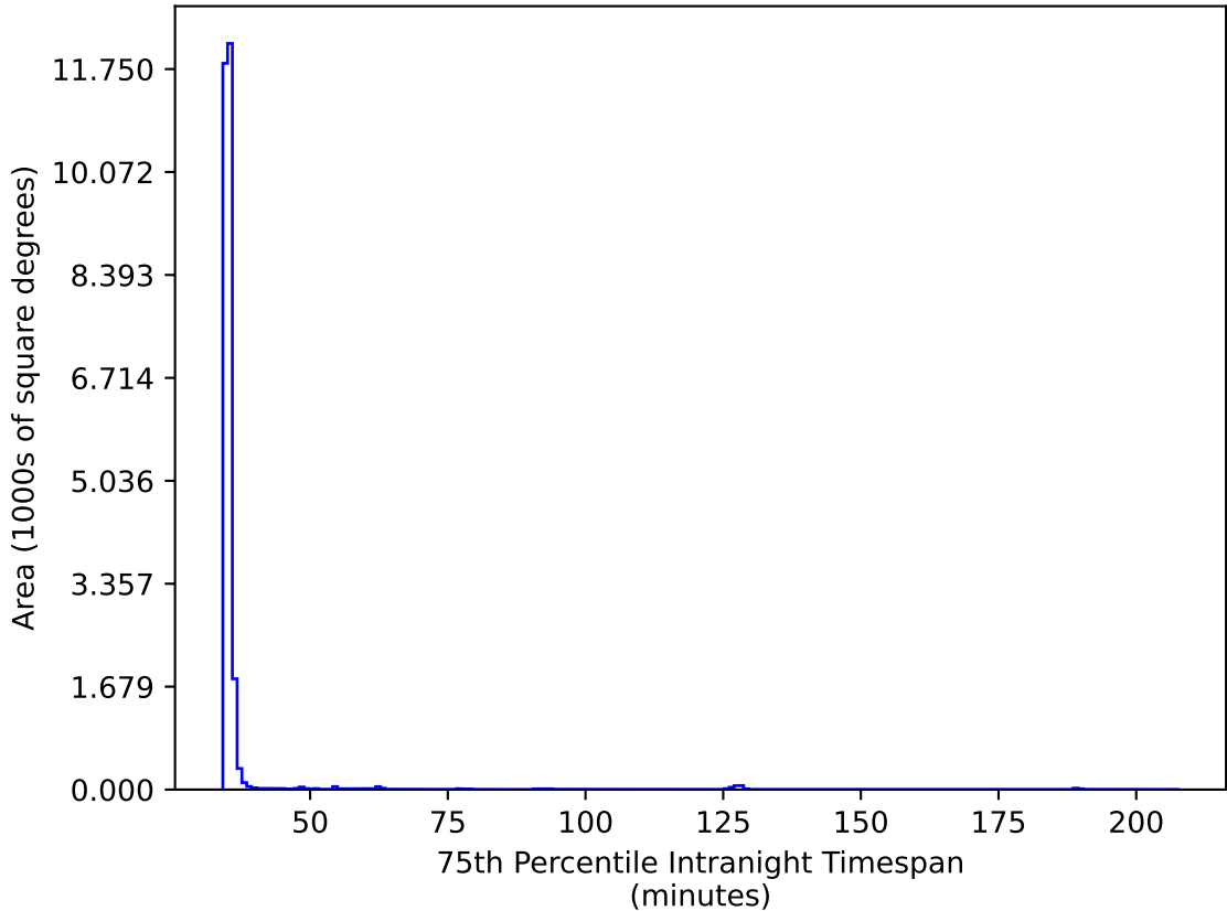
baseline_v3.2_10yrs All sky iz bands: 75th Percentile Intranight Timespan
