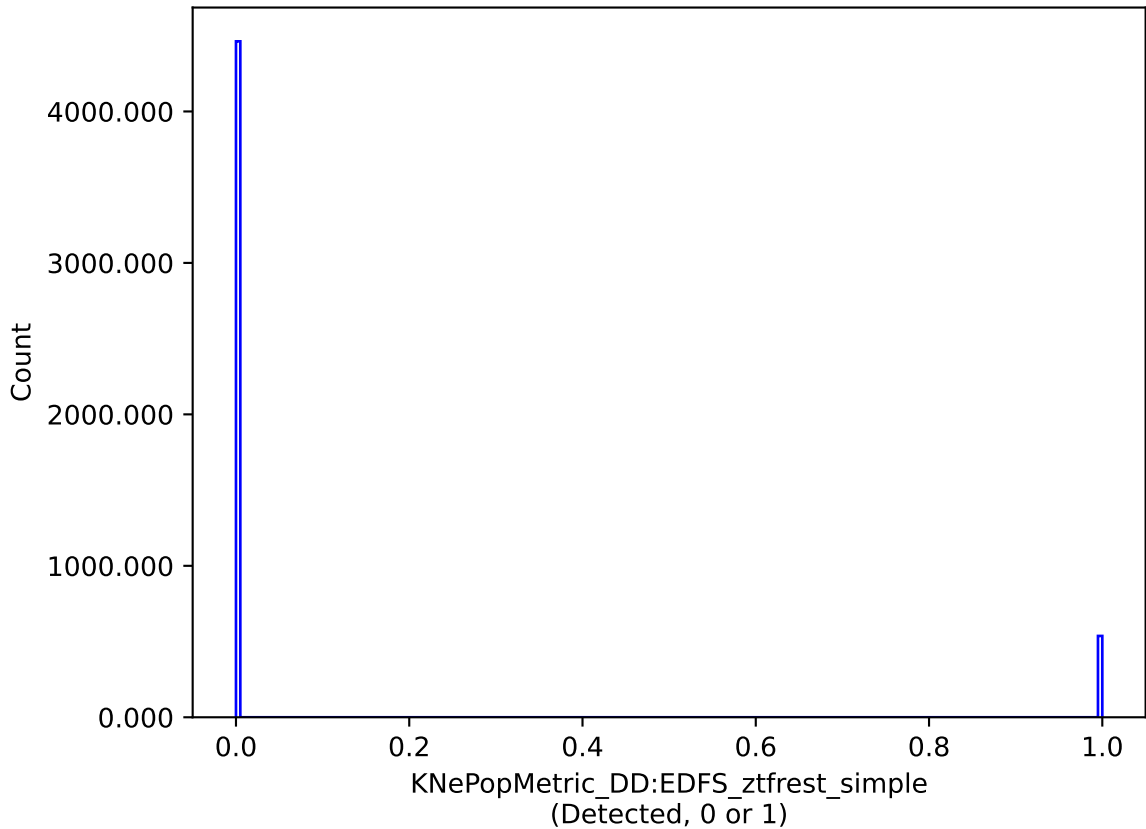
baseline_v3.2_10yrs DD:EDFS: KNePopMetric_DD:EDFS_ztfrest_simple
