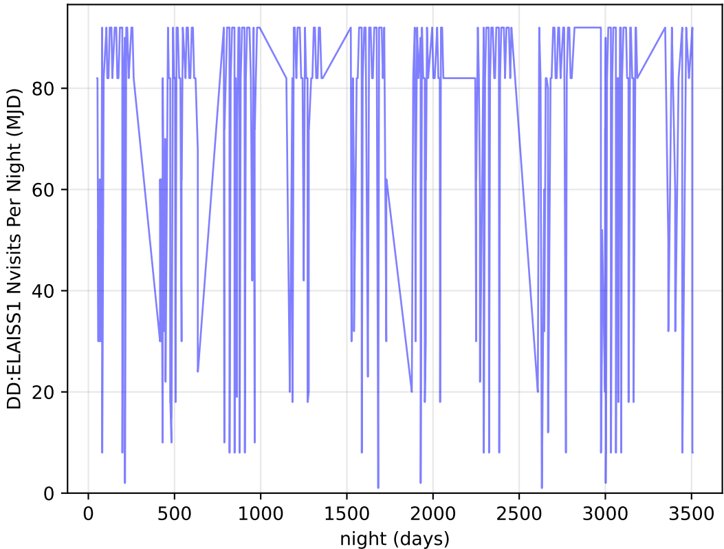
baseline_v3.2_10yrs all bands: DD:ELAISS1 Nvisits Per Night
