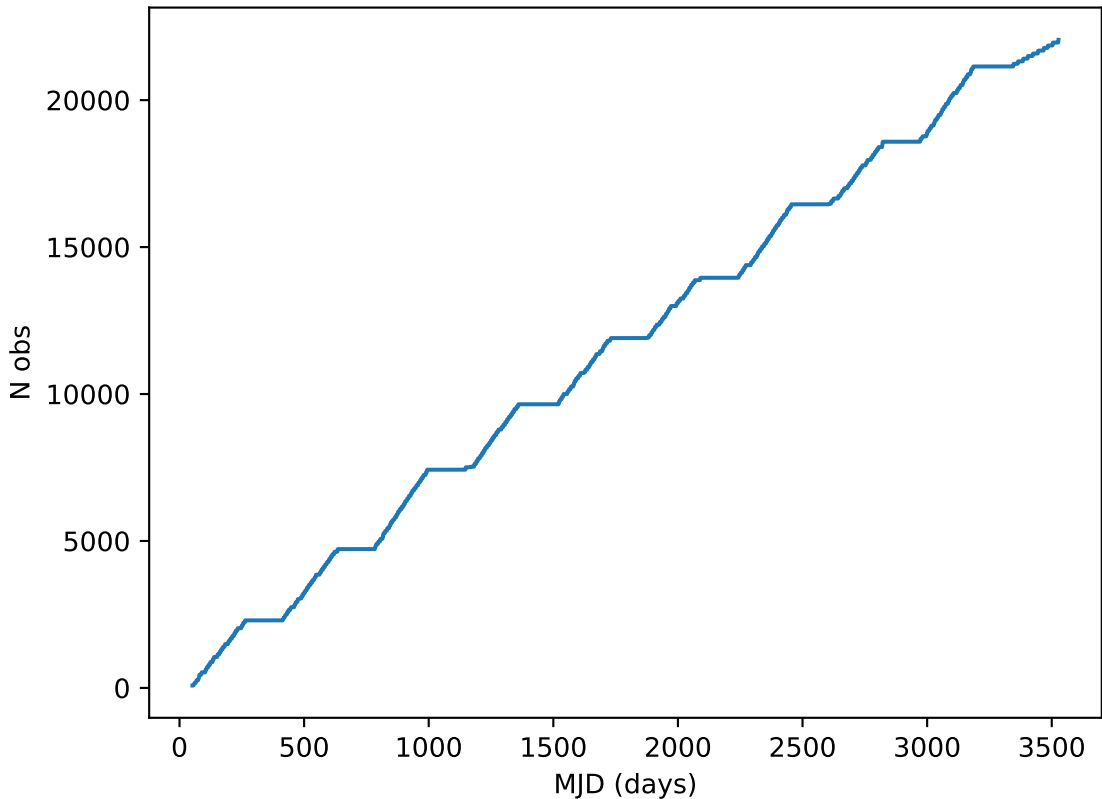
baseline_v3.2_10yrs all bands: DD:ELAISS1 Cumulative NVisits
