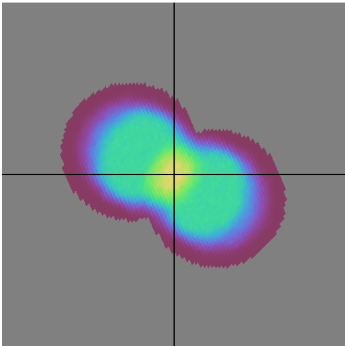
baseline_v3.2_10yrs z band: DD:EDFS NVisits
