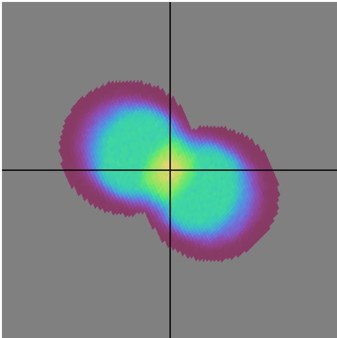
baseline_v3.2_10yrs r band: DD:EDFS NVisits
