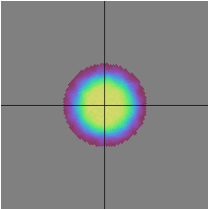
baseline_v3.2_10yrs z band: DD:ECDFS NVisits
