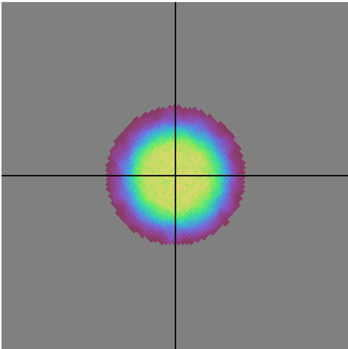
baseline_v3.2_10yrs y band: DD:ECDFS NVisits
