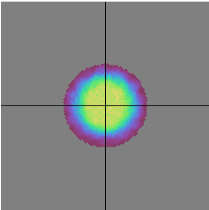
baseline_v3.2_10yrs u band: DD:ECDFS NVisits
