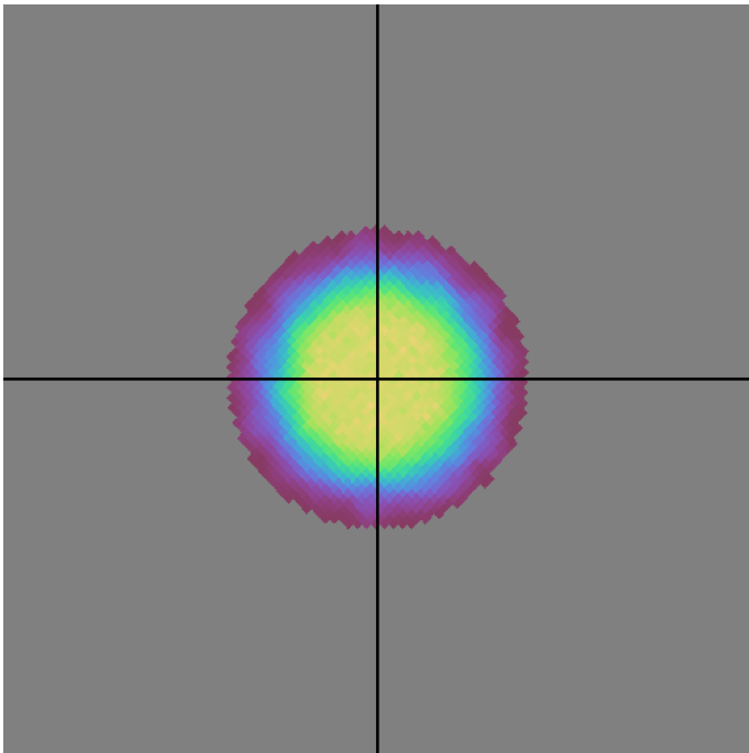
baseline_v3.2_10yrs i band: DD:ECDFS NVisits
