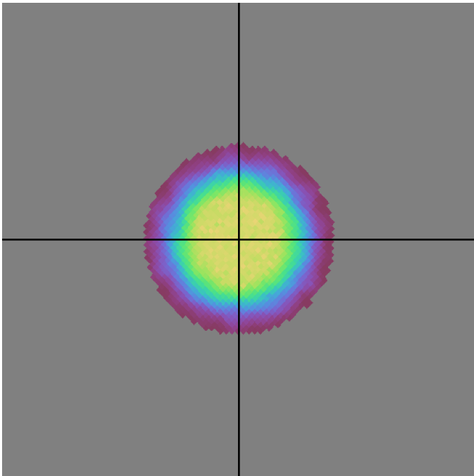
baseline_v3.2_10yrs g band: DD:ECDFS NVisits
