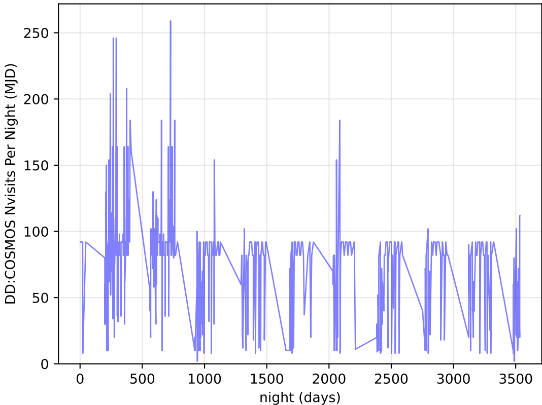
baseline_v3.2_10yrs all bands: DD: COSMOS Nvisits Per Night
