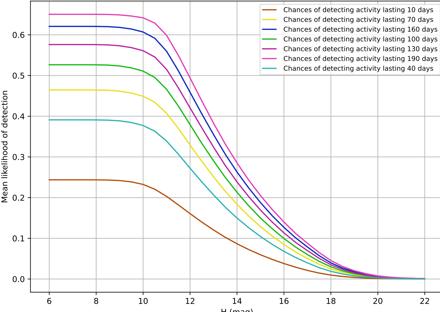
baseline_v3.0_10yrs OCC_r5
