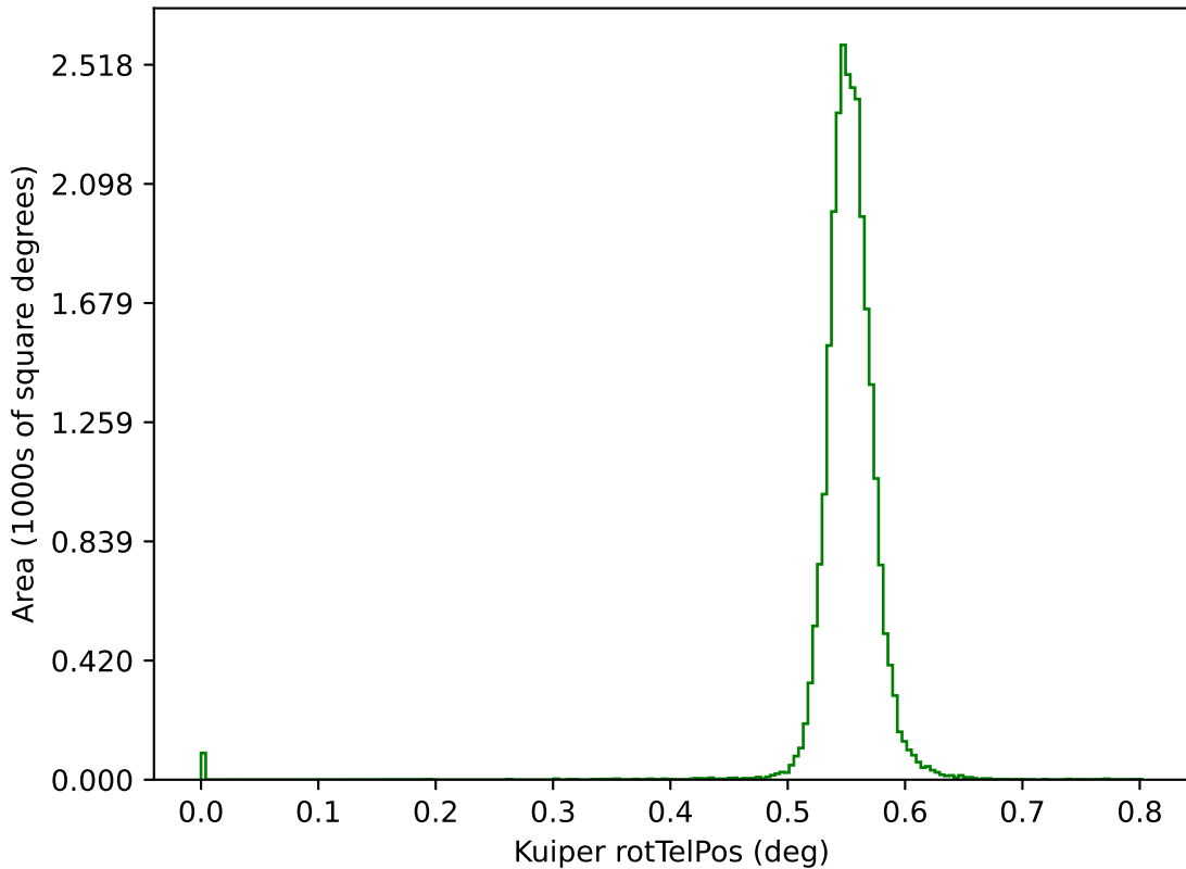
baseline_v3.0_10yrs g: Kuiper rotTelPos
