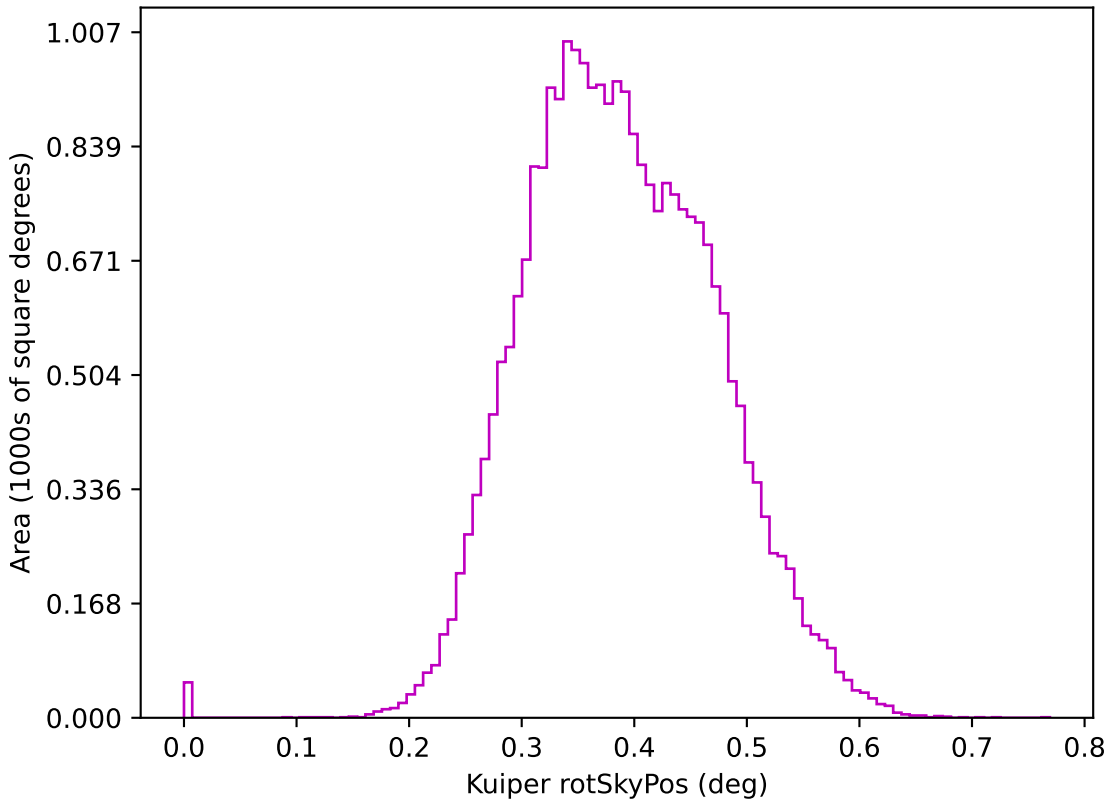
baseline_v3.0_10yrs z: Kuiper rotSkyPos
