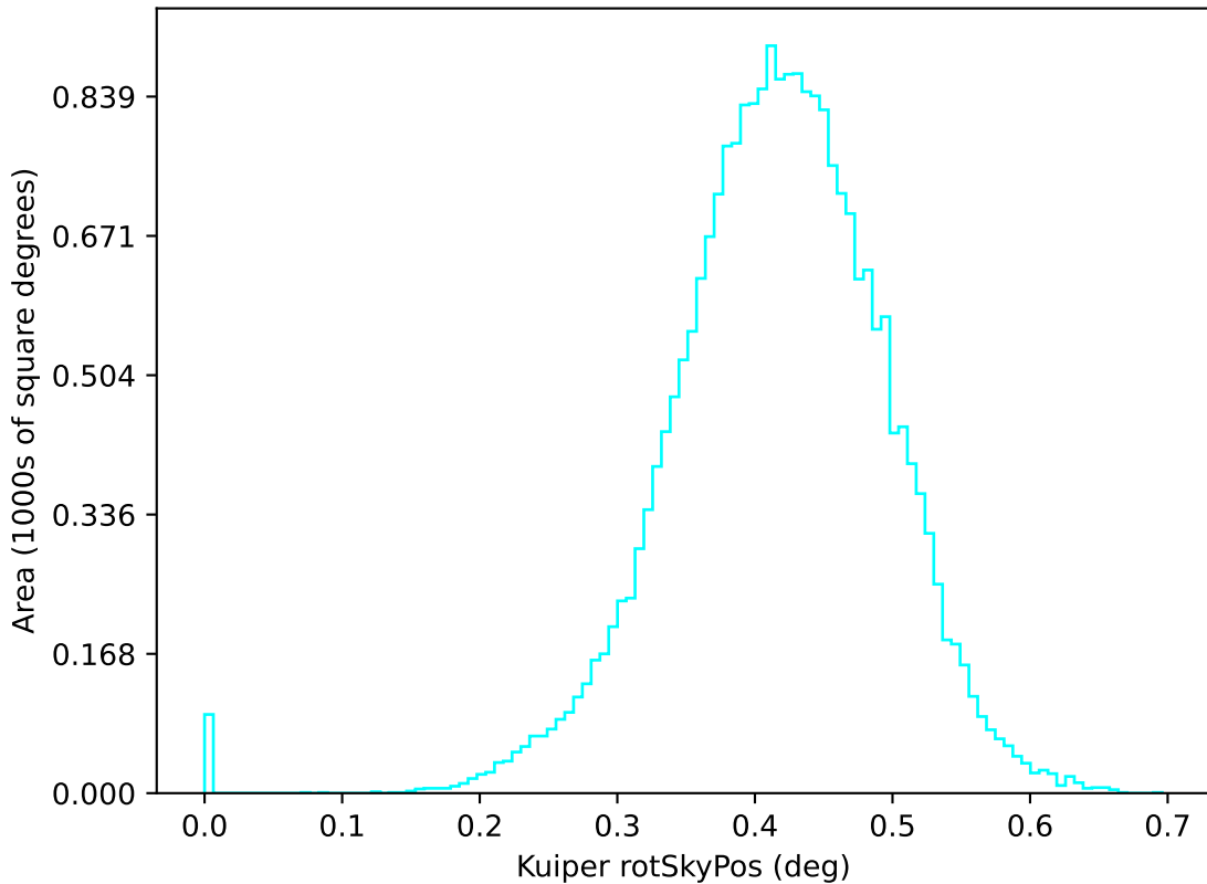
baseline_v3.0_10yrs u: Kuiper rotSkyPos
