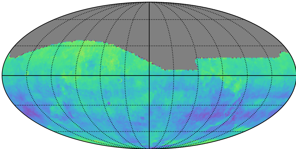
baseline_v3.0_10yrs i: Kuiper rotSkyPos
