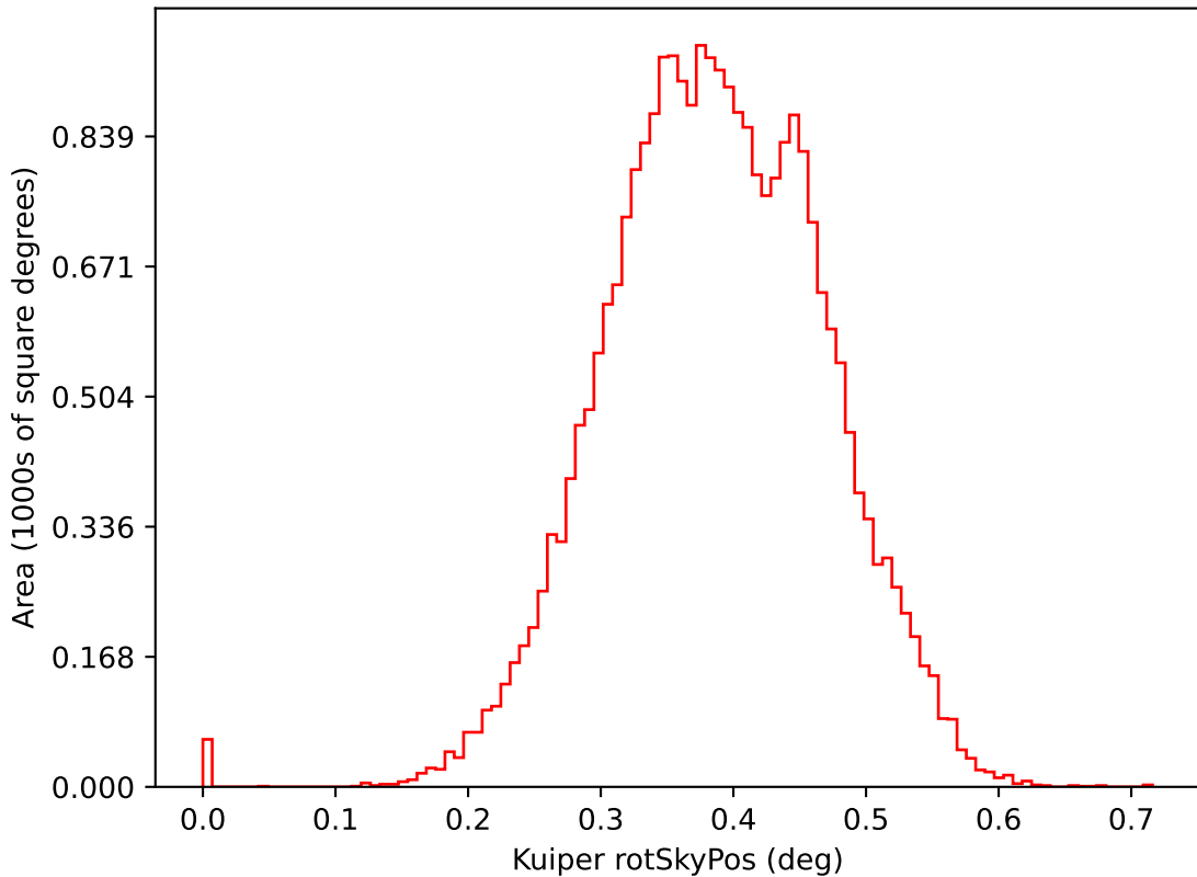
baseline_v3.0_10yrs i: Kuiper rotSkyPos
