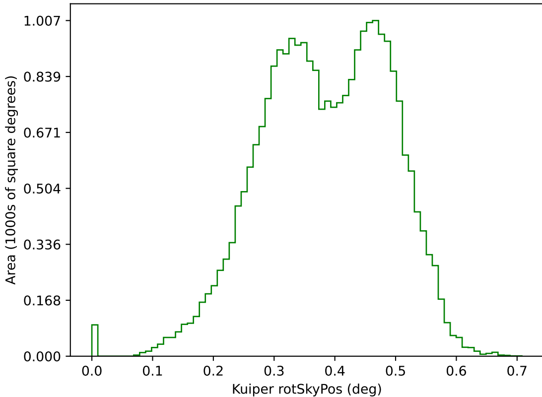
baseline_v3.0_10yrs g: Kuiper rotSkyPos
