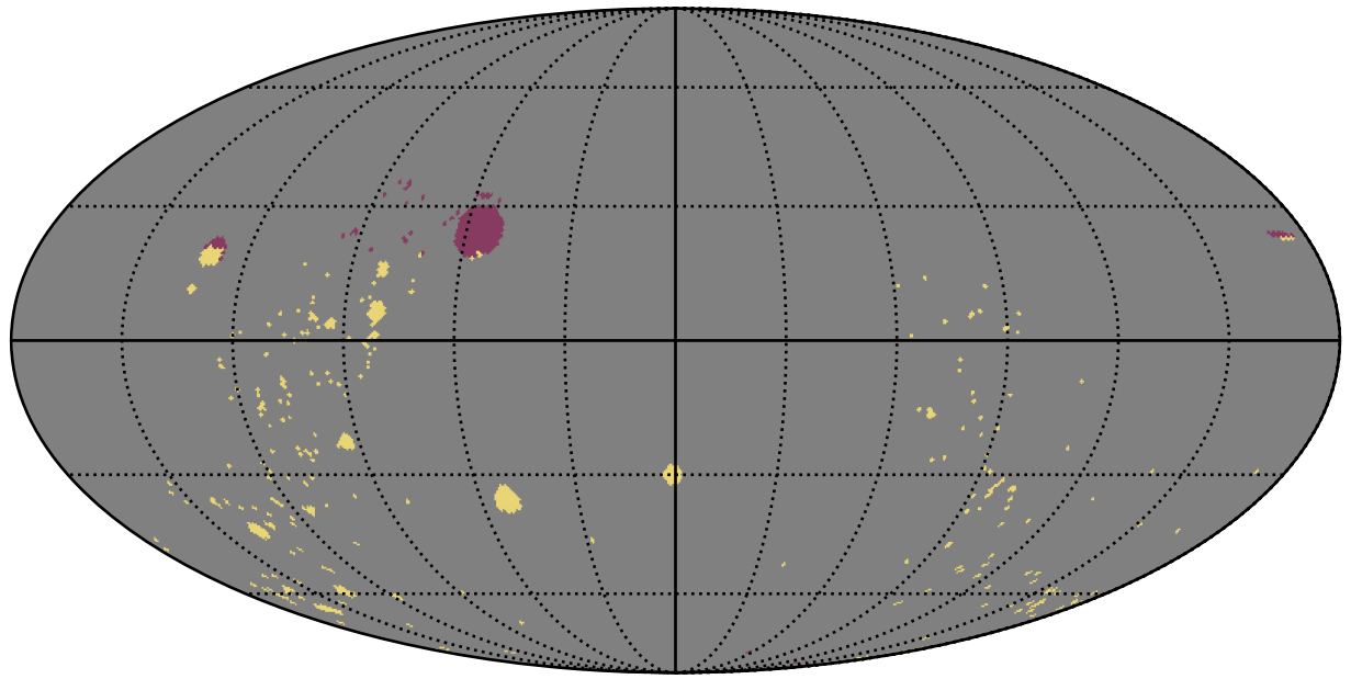
baseline_v3.0_10yrs : GalplaneFootprintMetric_open_clusters_map_Tau_46_5
