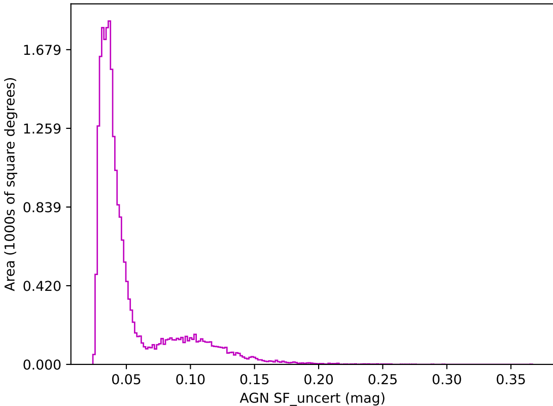
baseline_v3.0_10yrs z band: AGN SF_uncert
