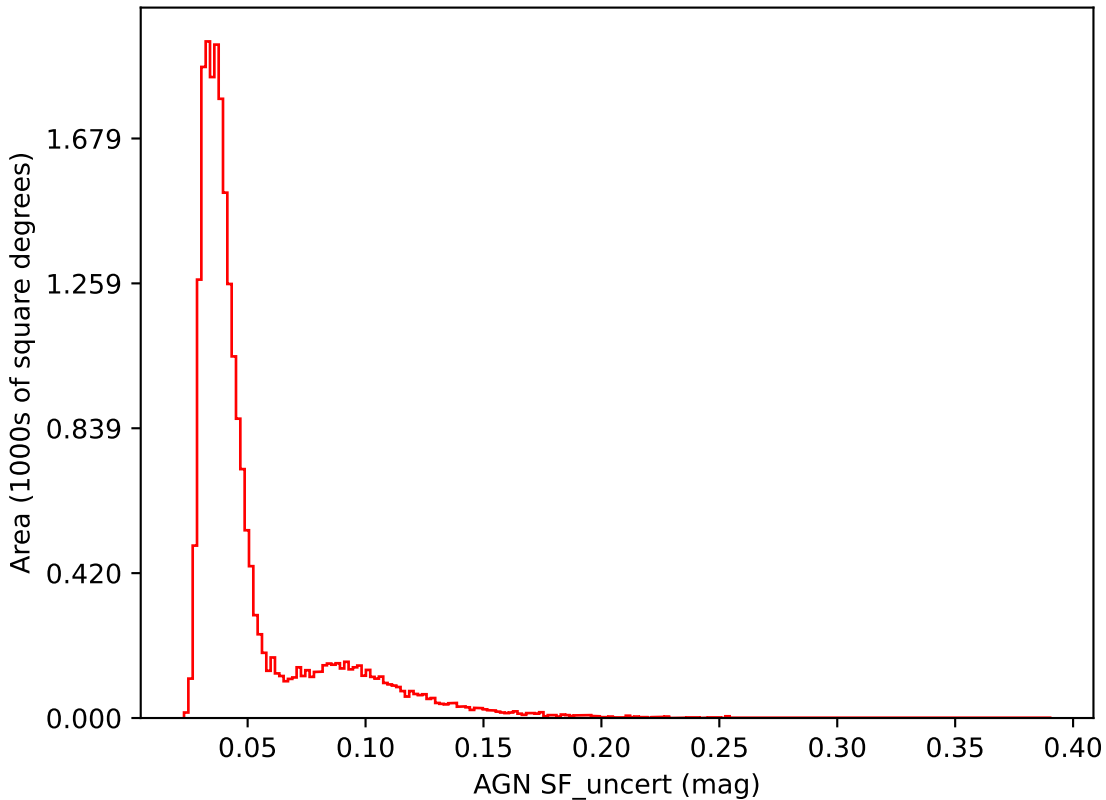
baseline_v3.0_10yrs i band: AGN SF_uncert
