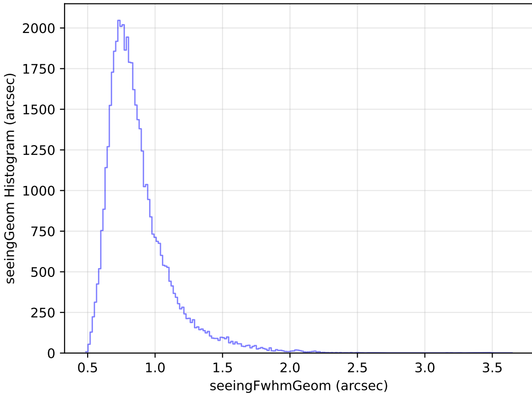
baseline_v3.0_10yrs Yr 1 y band: seeingGeom Histogram
