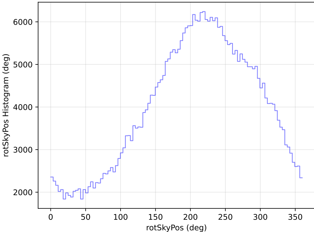
baseline_v3.0_10yrs WFD y band: rotSkyPos Histogram
