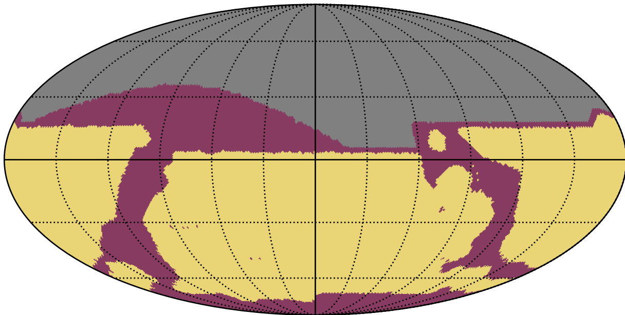
baseline_v3.0_10yrs All sky: RapidRevisits
