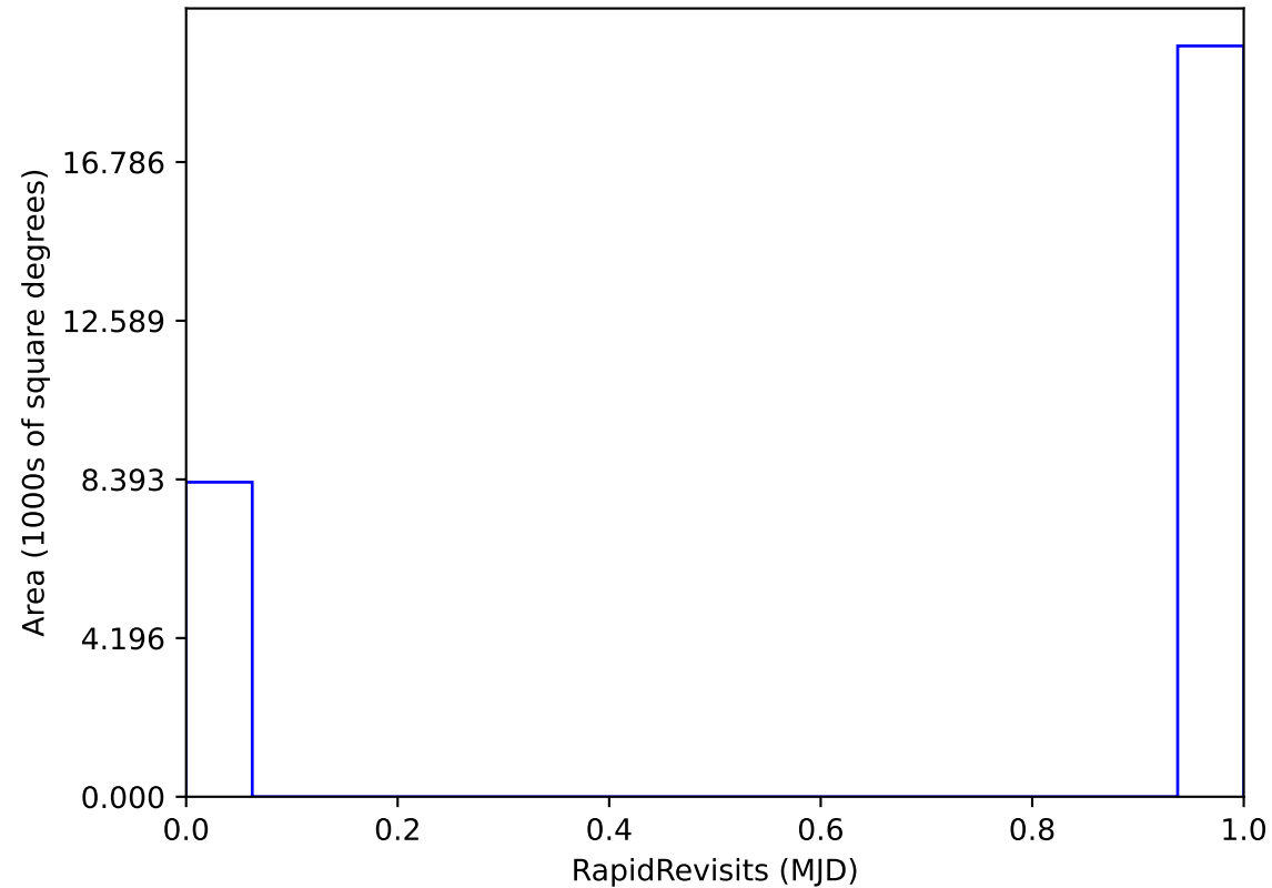
baseline_v3.0_10yrs All sky: RapidRevisits
