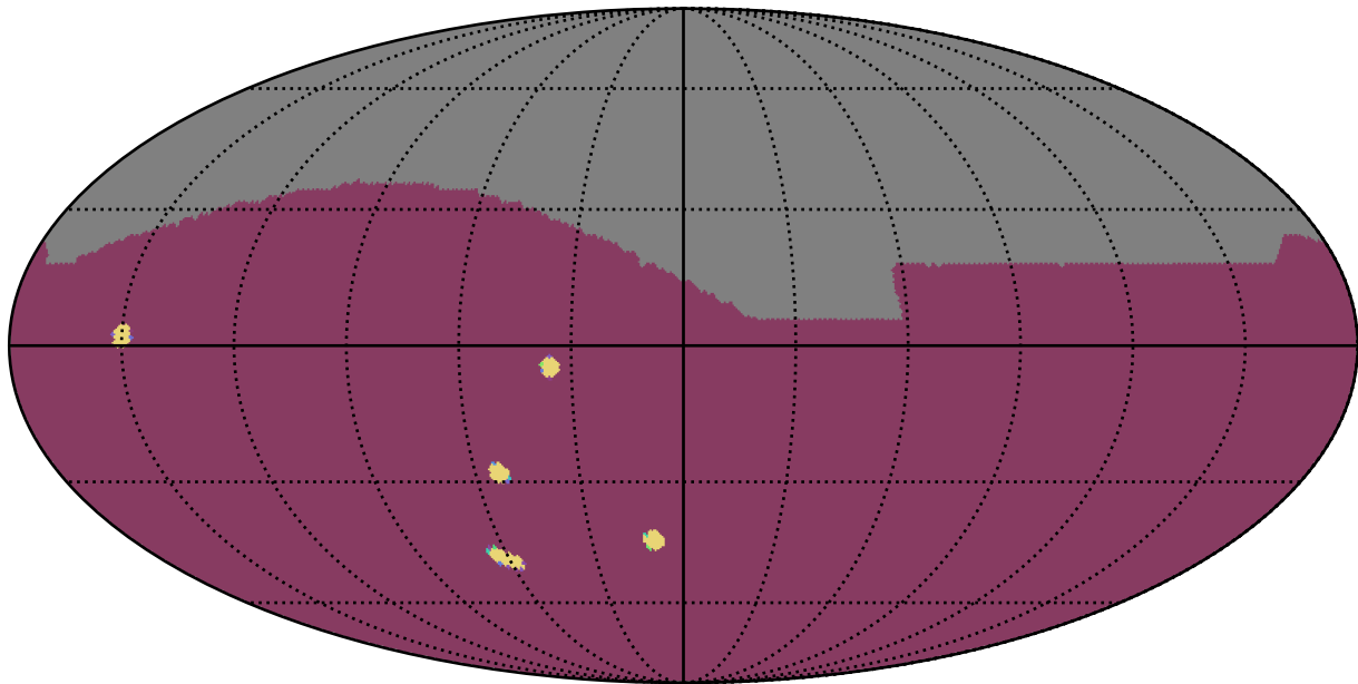
baseline_v3.0_10yrs All sky: NumberOfQuickRevisits
