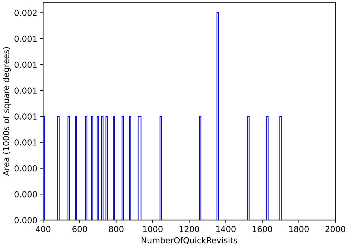
baseline_v3.0_10yrs All sky: NumberOfQuickRevisits
