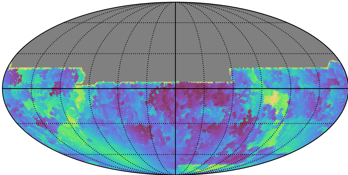
baseline_v3.0_10yrs All sky y band: Min solarElong
