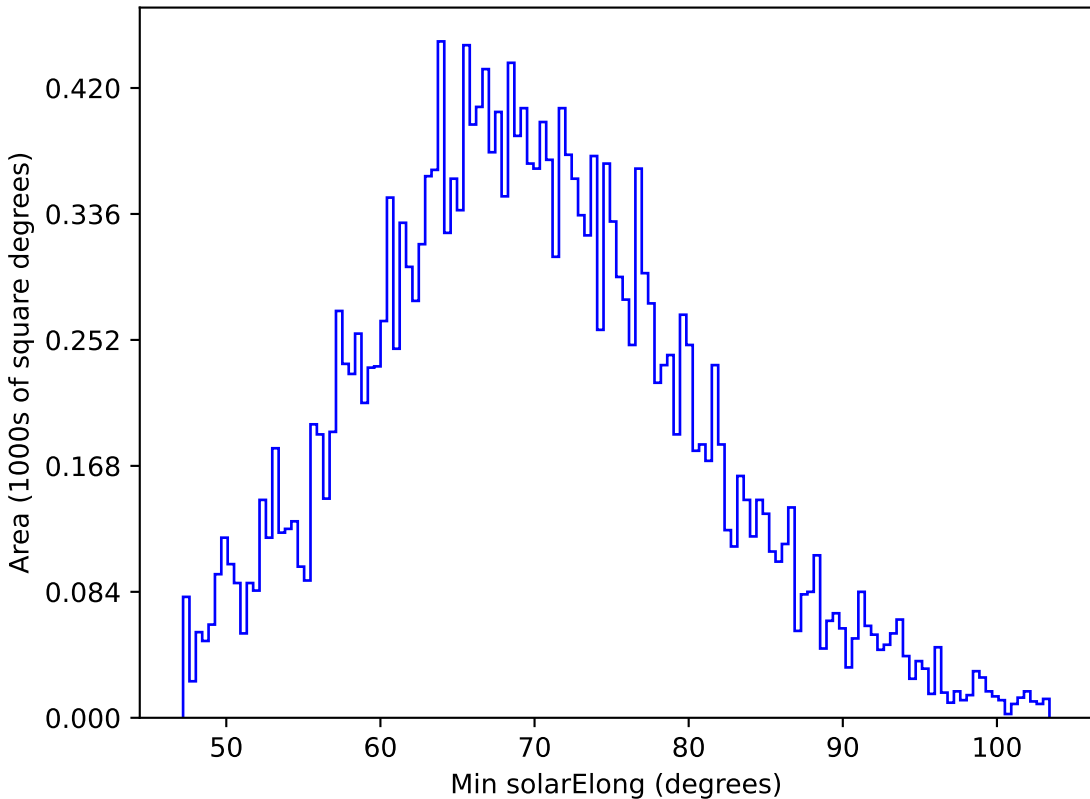
baseline_v3.0_10yrs All sky y band: Min solarElong
