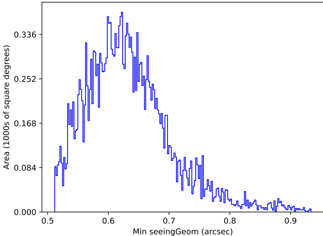
baseline_v3.0_10yrs Yr 1 y band: Min seeingGeom
