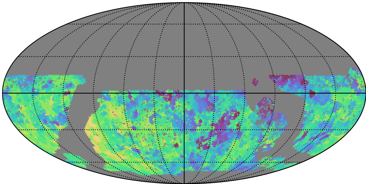
baseline_v3.0_10yrs WFD y band: Min saturation_mag
