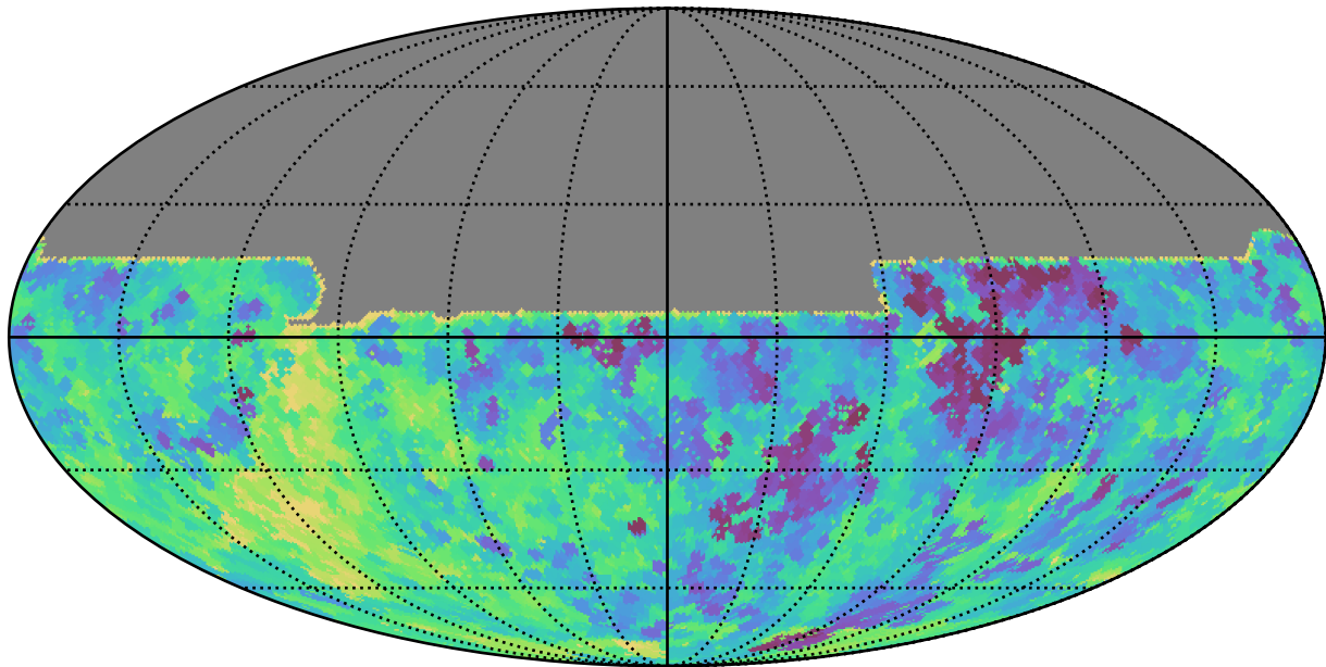
baseline_v3.0_10yrs All sky y band: Min saturation_mag
