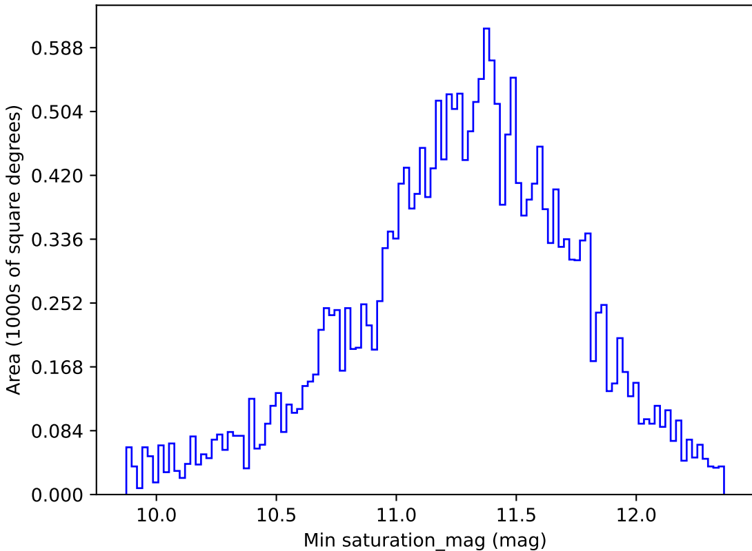
baseline_v3.0_10yrs All sky y band: Min saturation_mag
