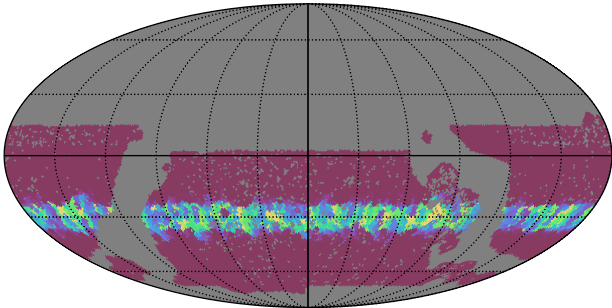
baseline_v3.0_10yrs WFD y band: Min normairmass
