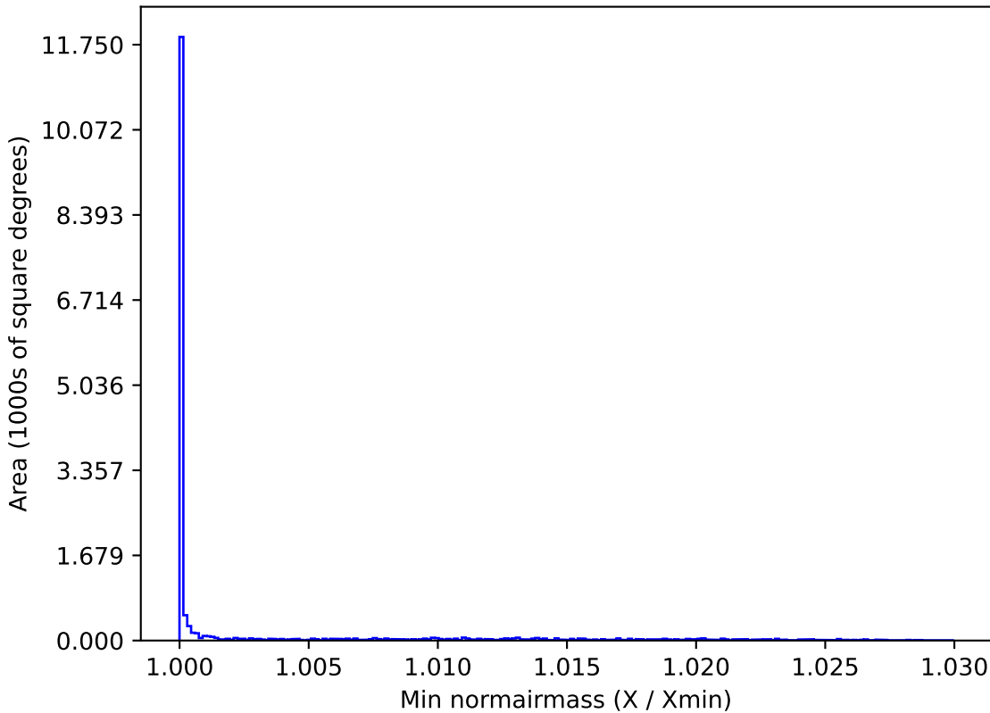
baseline_v3.0_10yrs WFD y band: Min normairmass
