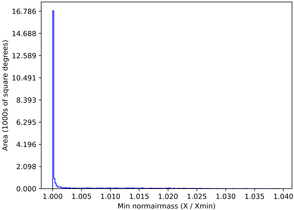
baseline_v3.0_10yrs All sky y band: Min normairmass
