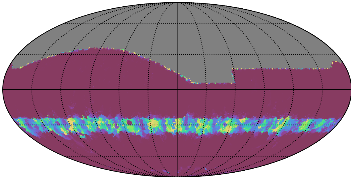
baseline_v3.0_10yrs All sky i band: Min normairmass
