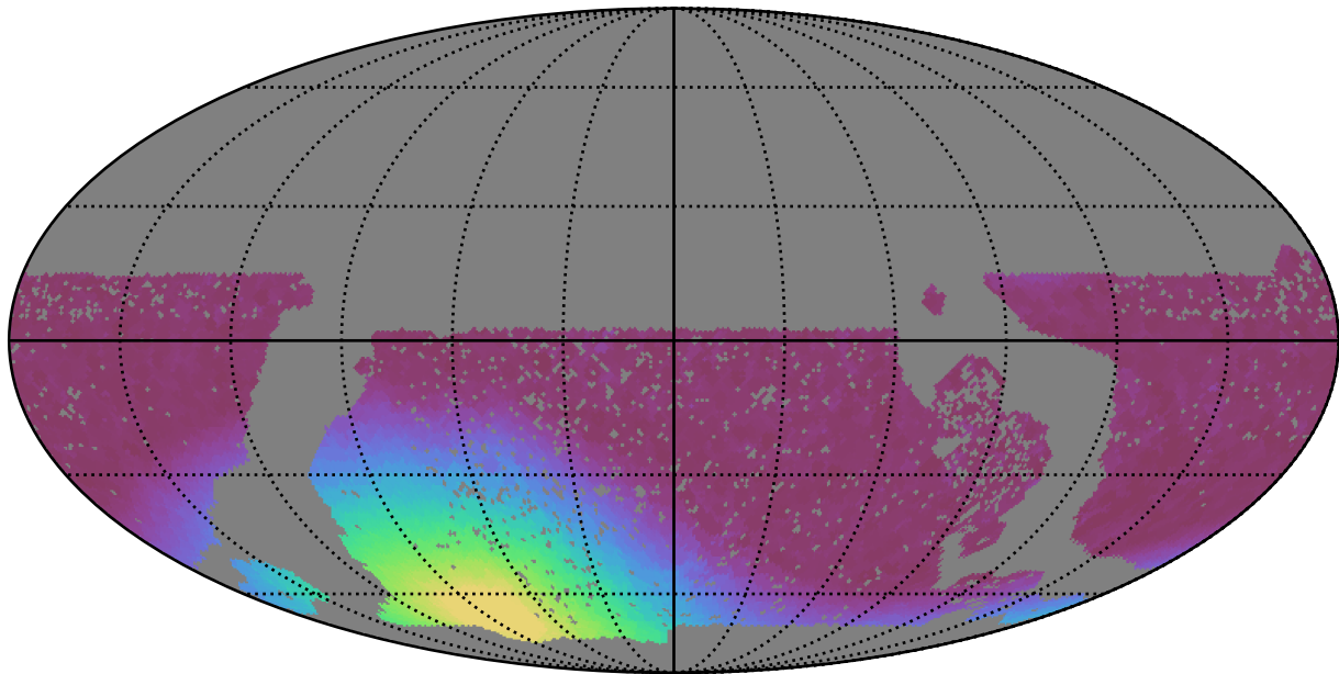
baseline_v3.0_10yrs WFD y band: Min moonDistance
