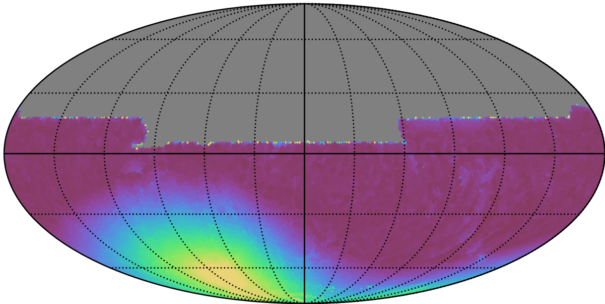
baseline_v3.0_10yrs All sky y band: Min moonDistance
