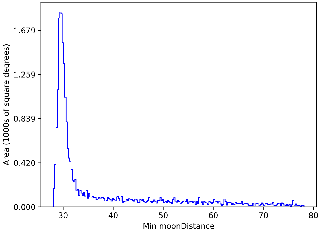
baseline_v3.0_10yrs All sky y band: Min moonDistance
